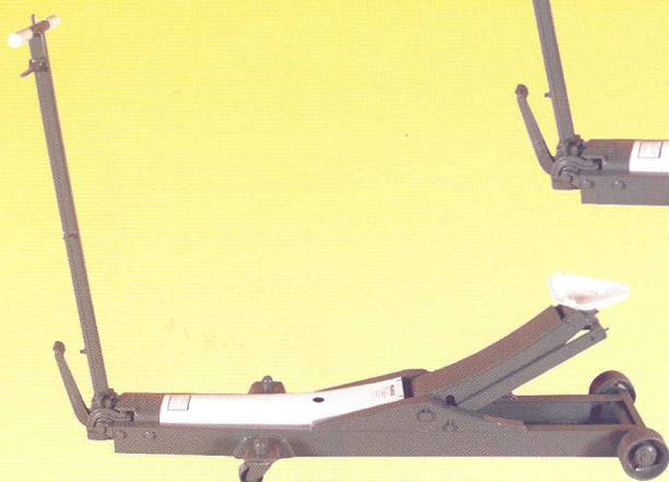
WA-72B
